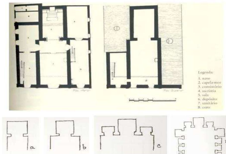
Figura 5 – Planta baixa da Igreja São Francisco de Paula
